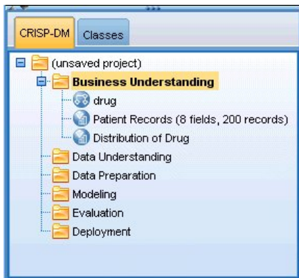
Figura 8. visualizzazione CRISP-DM
