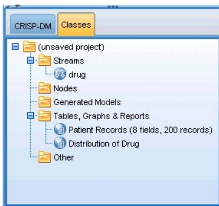
Figura 9. Vista Classi
